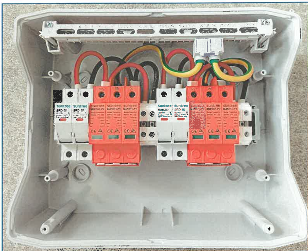
Obr. 4 - Vybavení rozváděče RS-FVE-DC2
